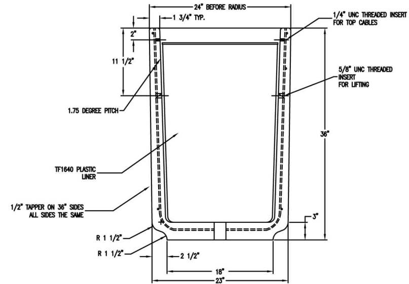
5 SECTION VIEW Scale: 1/8" = 1"
